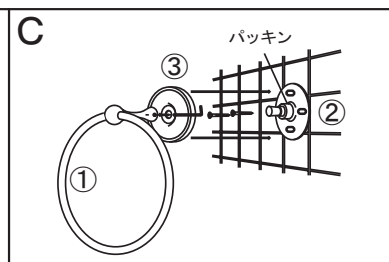
タオルリング取付参考図です。 商品によりイラストが異なりますので 各商品の取付参考にして下さい。
